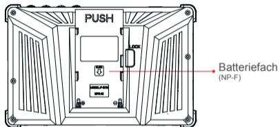
▼ Rückansicht
