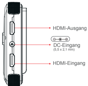
▼ Ansicht links
