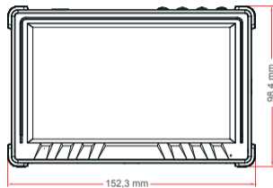
▼ Vorderansicht
